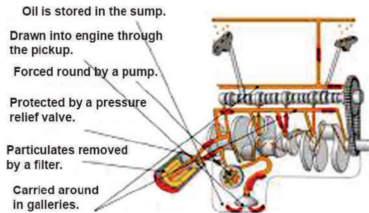
Fig. 2.1.2: Wet-sump type lubrication
