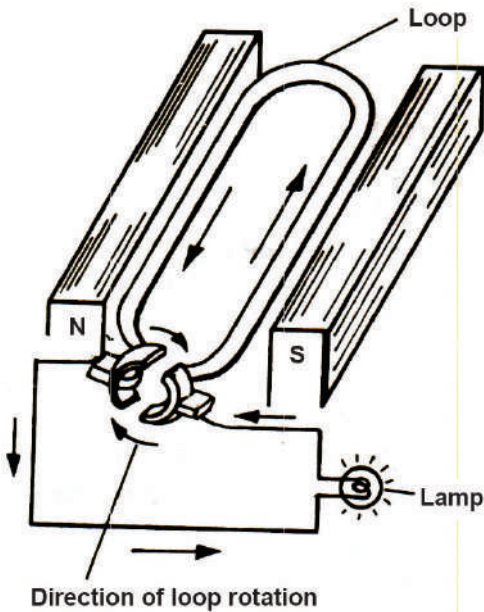
Fig. 6.2.4: Simple Generator
